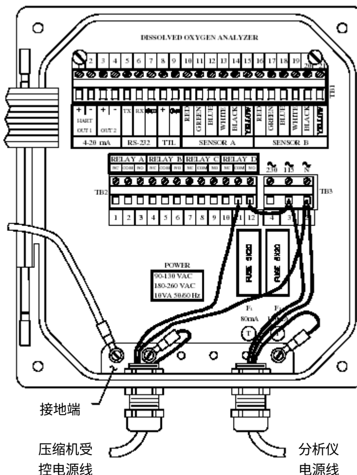
图 2-9 D53 分析仪与空气压缩机的接线
